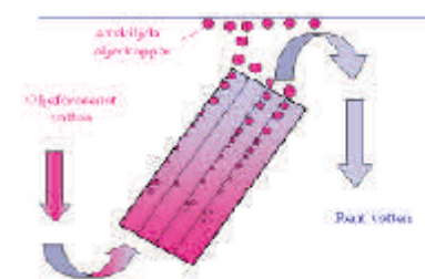
Principskiss av en koalesator. Små oljedroppar slås samman till större droppar som stiger till ytan och renat vatten kan avskiljas.
