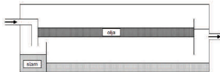
Principskiss av en gravimetrisk Klass II-oljeavskiljare
