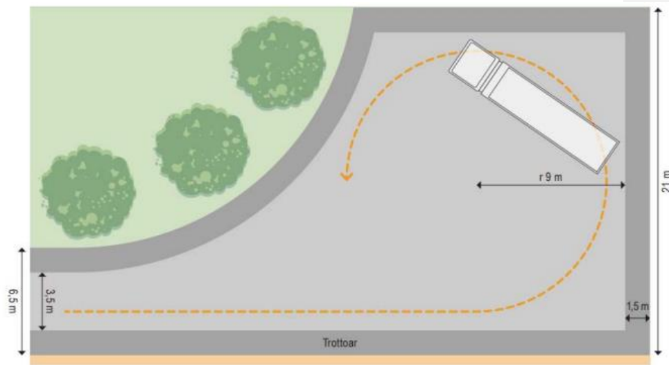
Figur 3 Måttangivelser för vändplan
