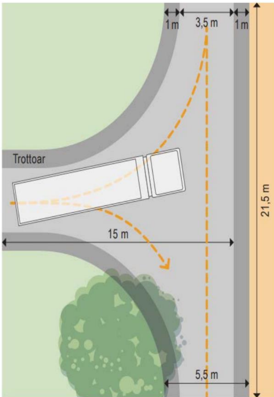
Figur 2 Måttangivelser för T-korsvändning
