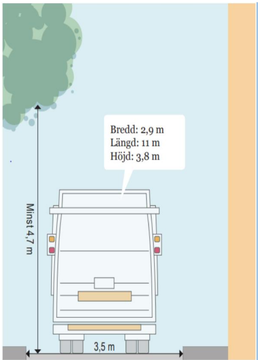
Figur 1 Måttangivelser för fordon
